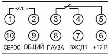
Рис. 6 Схема подключения ARCOM-TC-D44
